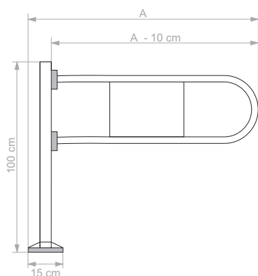
RAMIĘ DWUKIERUNKOWE Bi-directional gate arm
